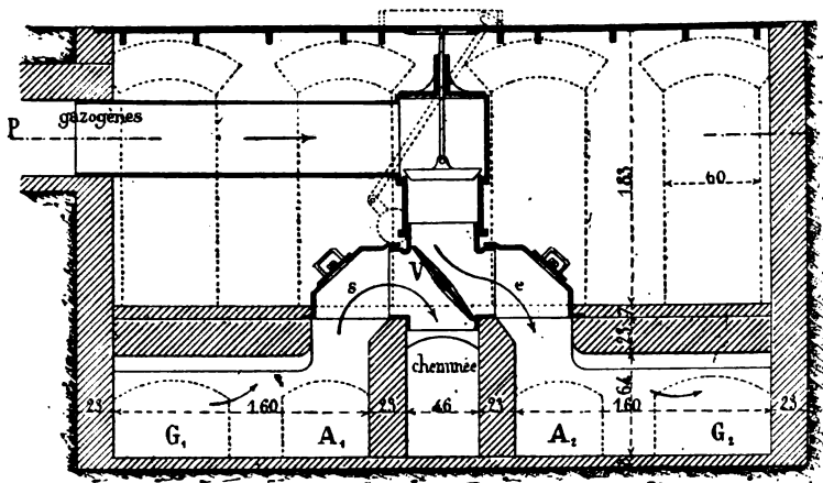
Coupe PQ
